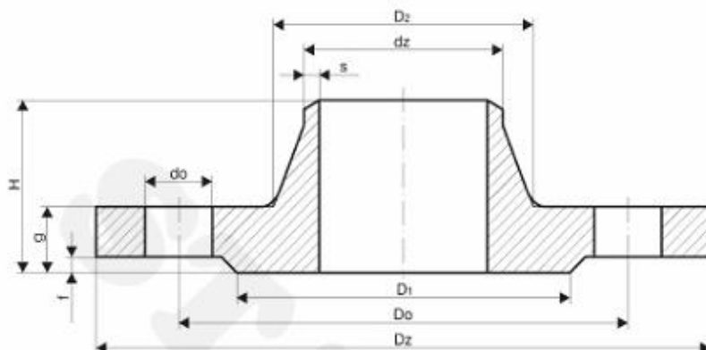
Neck flanges according to ANSI B16.5 kl. 150lbs
