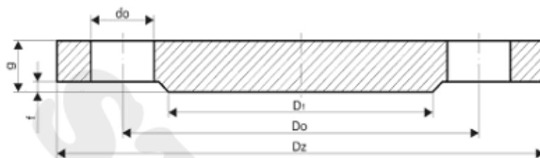
Blind flanges according to ANSI B16.5 kl. 150lbs
