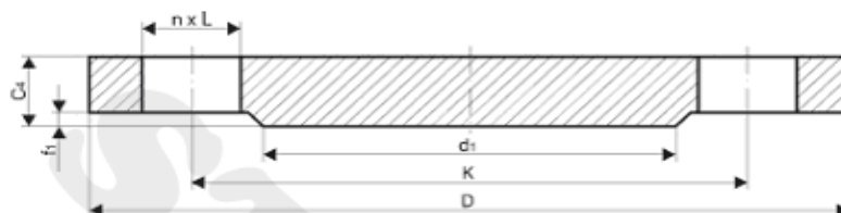
Blind flanges type 05 EN 1092-1:2001
