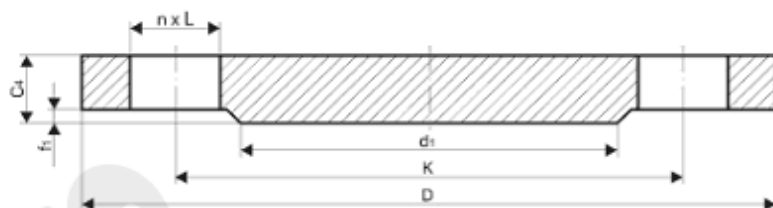
Blind flanges type 05 EN 1092-1:2001
